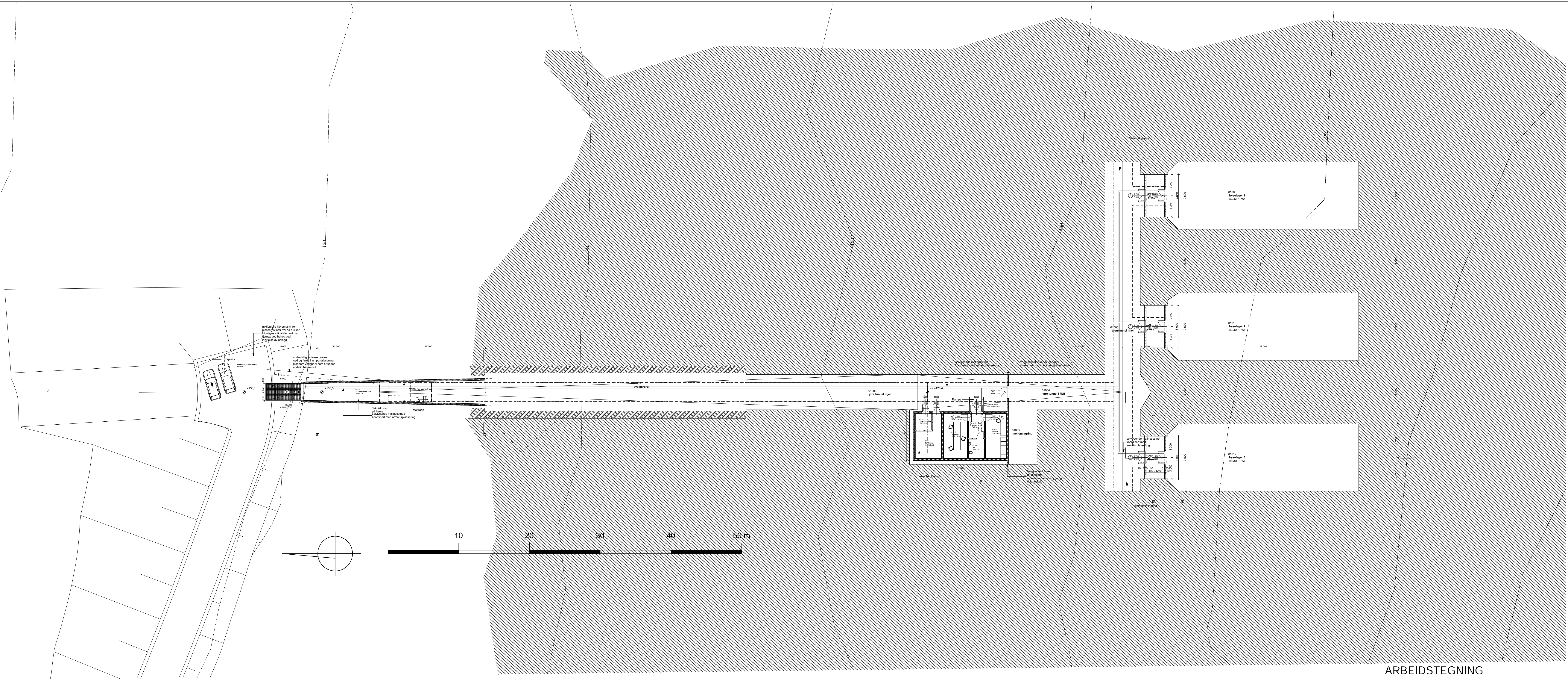
plan1 - hovedplan hele anlegget
